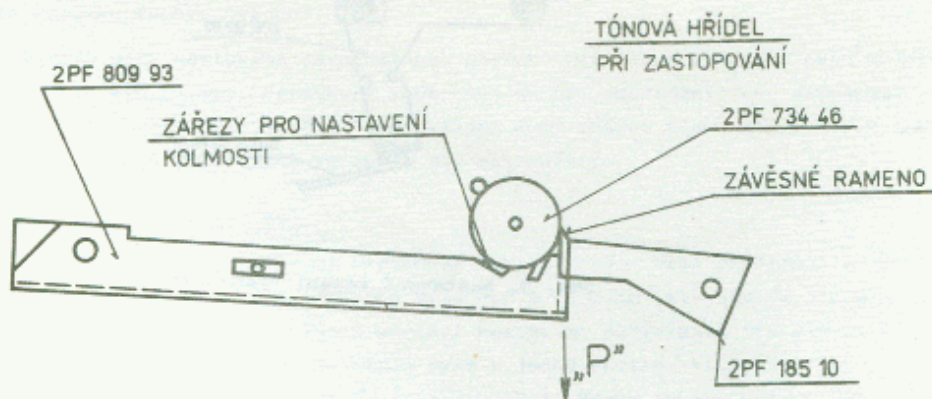
Obr. 5. Nastavení a kontrola tlaku přitlačné kladky
