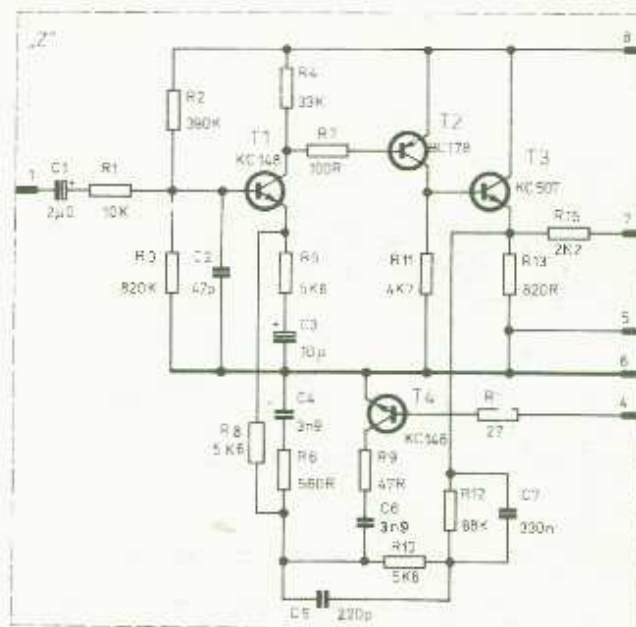
Obr. 23. Schéma záznamového zesilovače
