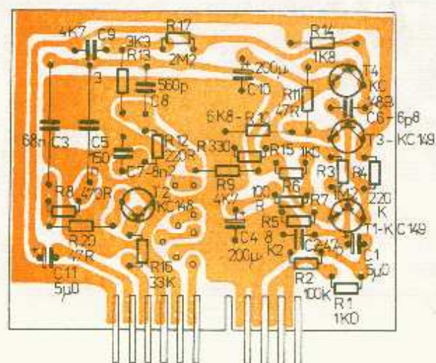
Obr. 19. Deska snímacího zesilovače (pohled ze strany směrůstek)
