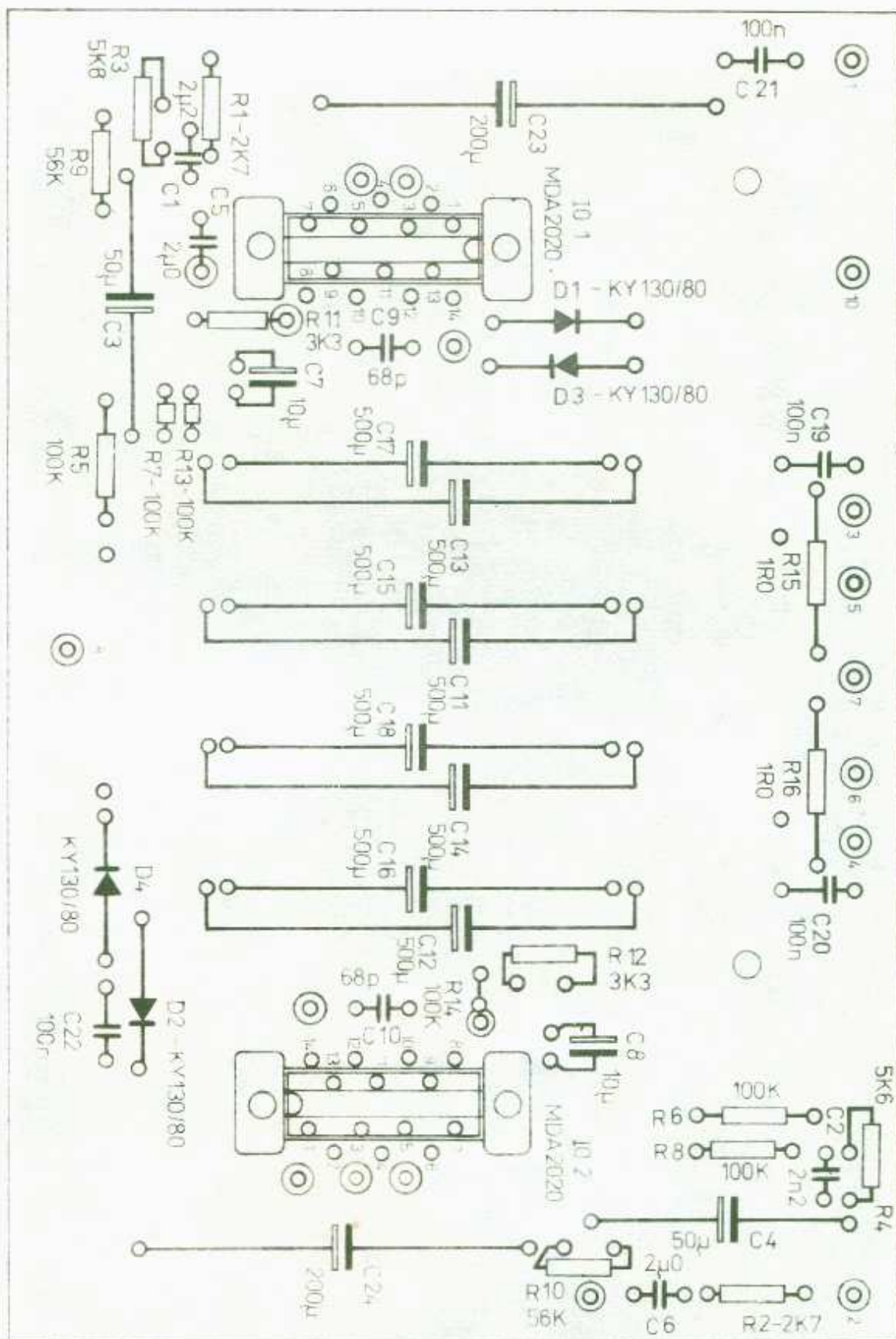
Obr. 39. Deska výkonového zesiluvce (pohled ze strany 10 "A")
