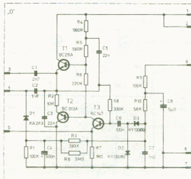
Obr. 28. Schéma zapojení oscilátoru
