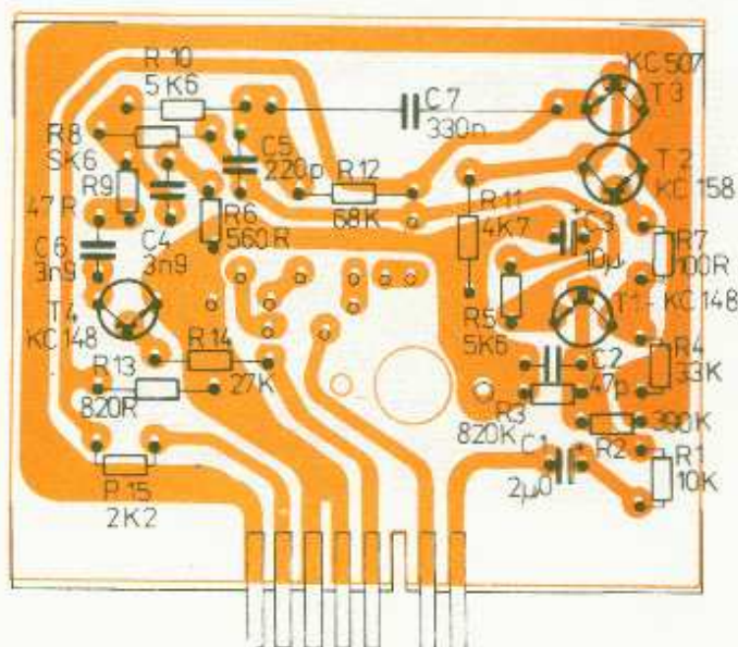
Obr. 25. Deska záznamového zesilovače (pohled ze strany spojů)
