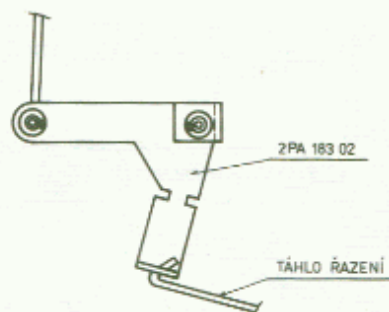
Obr. 3. Nastavení řazení rychlosti
