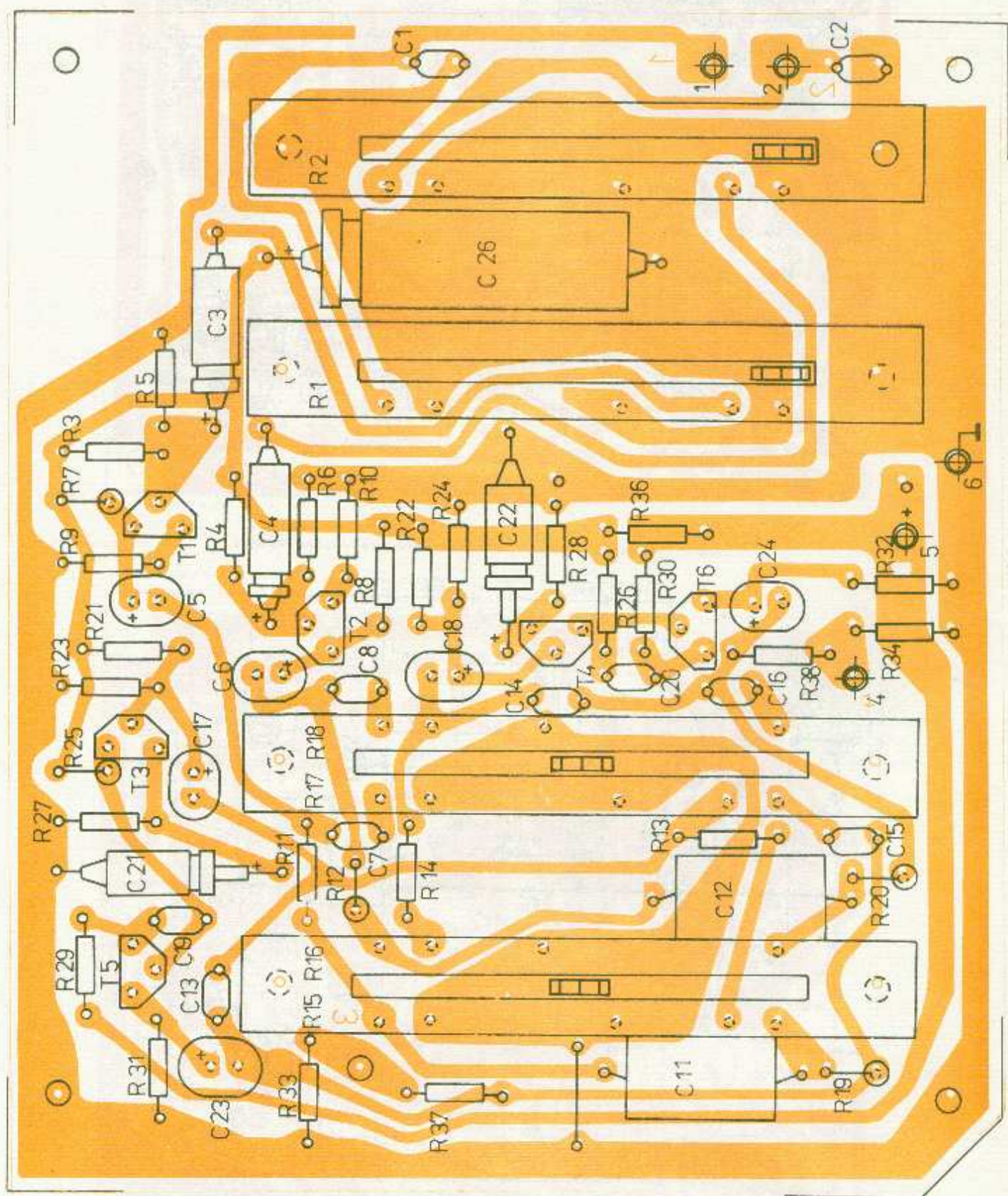
Obr. 16. Deska tónových korekcí (pohľad ze strany součástek)
