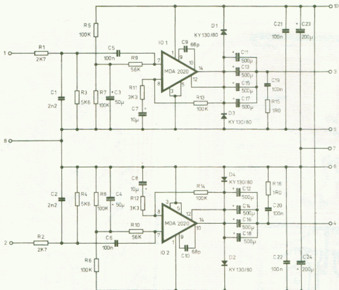
Obr. 38. Schéma zapojení výkonového zesilovače
