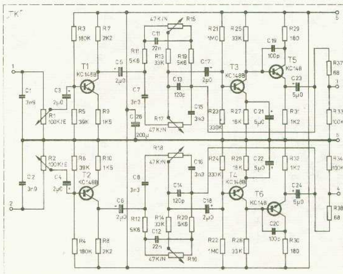
Obr. 15. Schéma tónových korekcí
