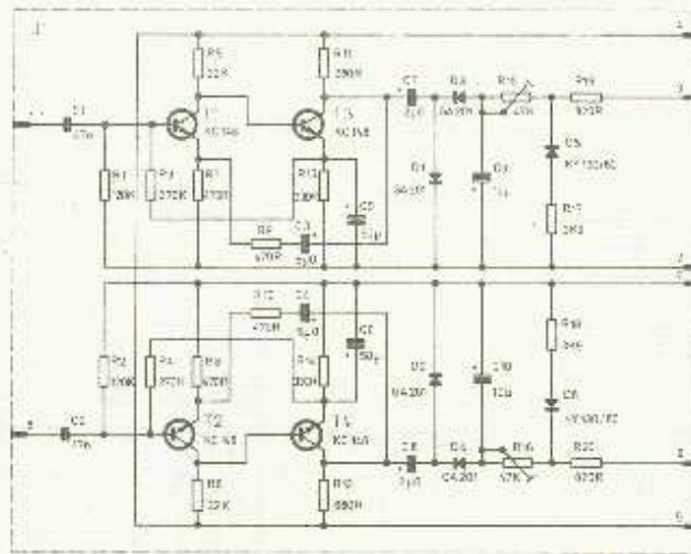
Obr. 31. Schéma zesilovače pro indikátory
