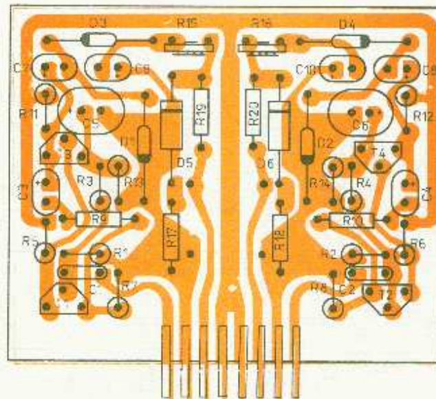
Obr. 32. Deska zesilovače pro indikátory (pohled ze strany součástek)
