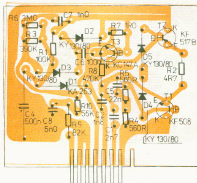
Obr. 30. Deska oscilátoru (pohled ze strany spojů)
