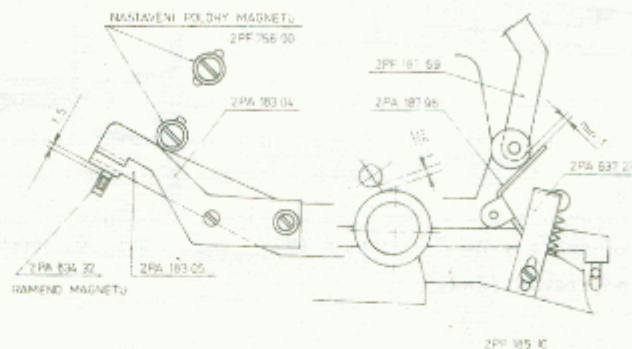
Obr. 6. Nastavení a kontrola funkce "stop"
