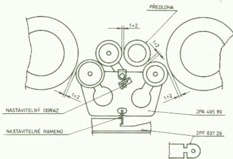
Obr. 2. Nastavení převíjecích kol
