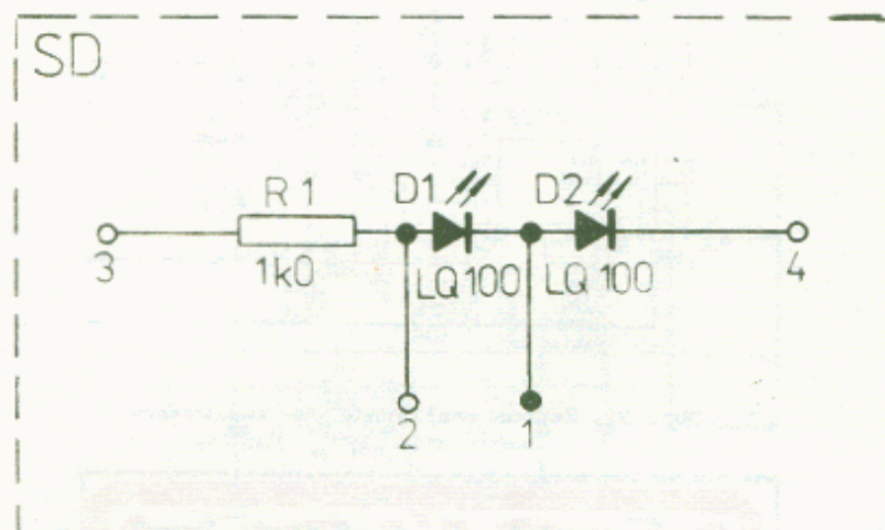
Obr. 34. Schéma desky světelných diod
