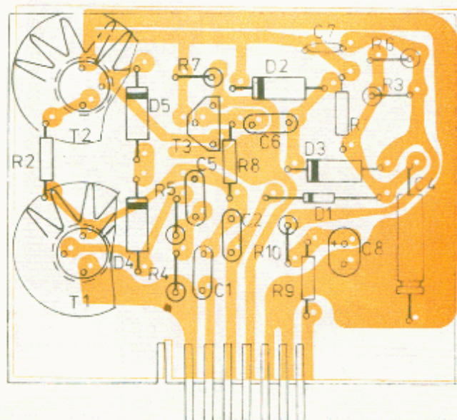
Obr. 29. Deska oscilátoru (pohled ze strany součástek)
