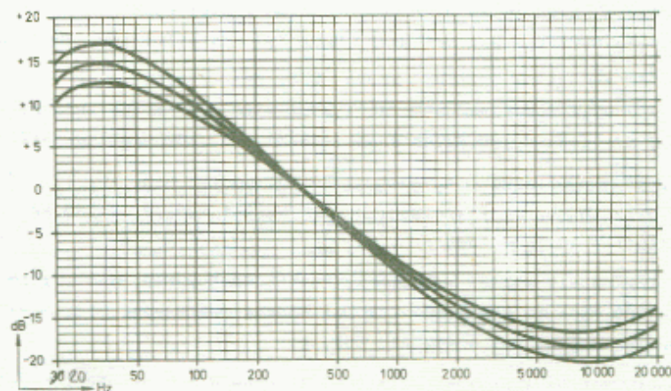
Obr. 22. Kmitočtová charakteristika SZ pro "v = 19"
