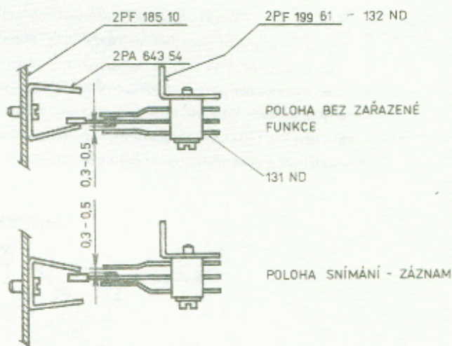
Obr. 9. Nastavení a kontrola pérového svazku
