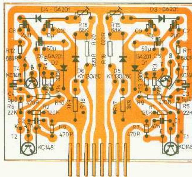
Obr. 33. Deska zesilovače pro indikátory (pohled ze strany spojů)
