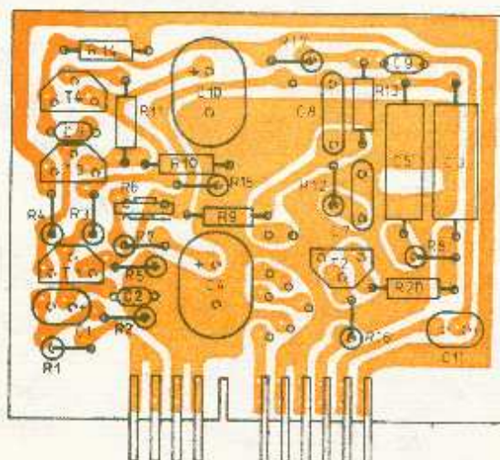
Obr. 19. Deska snímacího zesilovače (pohled ze strany směrůstek)
