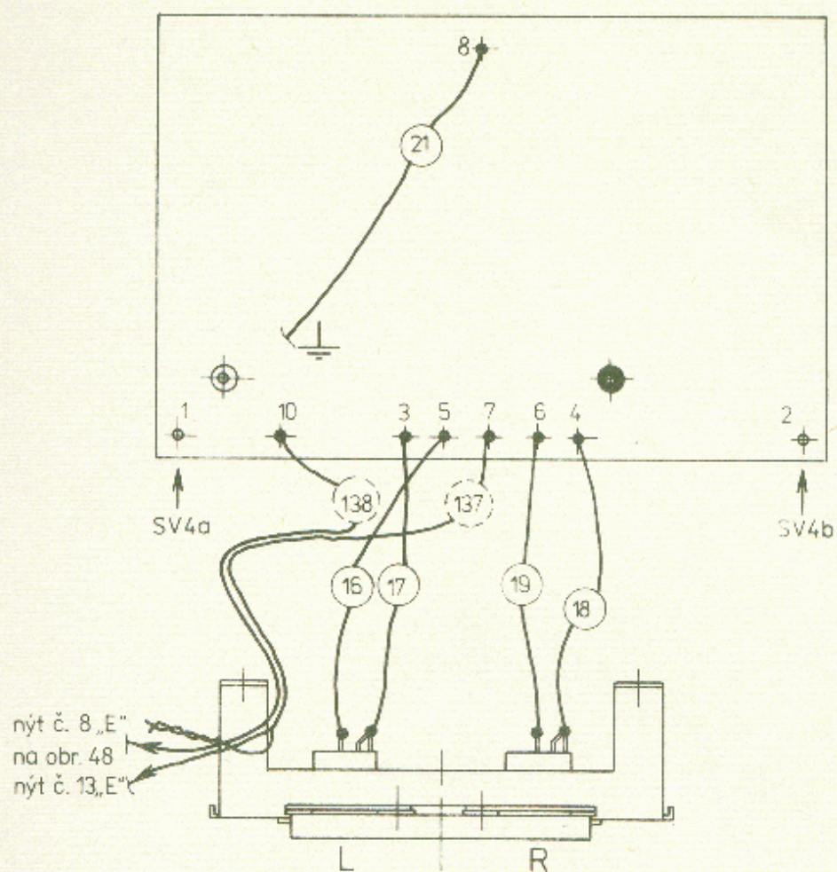
Obr. 50. Výkonový zesilovač zapojený
