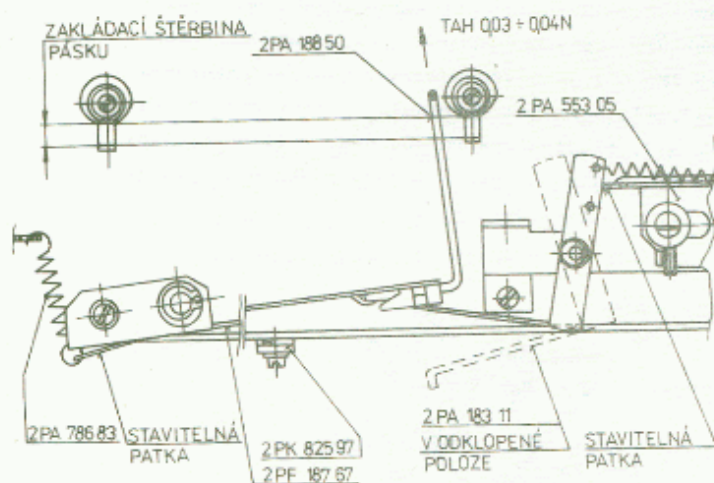
Obr. 8. Nastavení a kontrola vypínání funkce při převinutí a přetržení pásku
