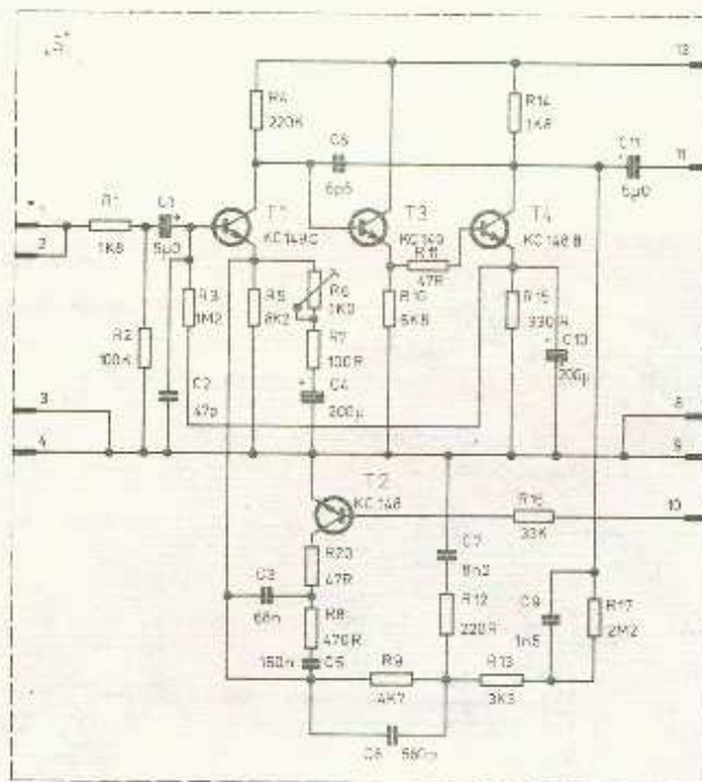
Obr. 18. Schéma snímacího zesilovače
