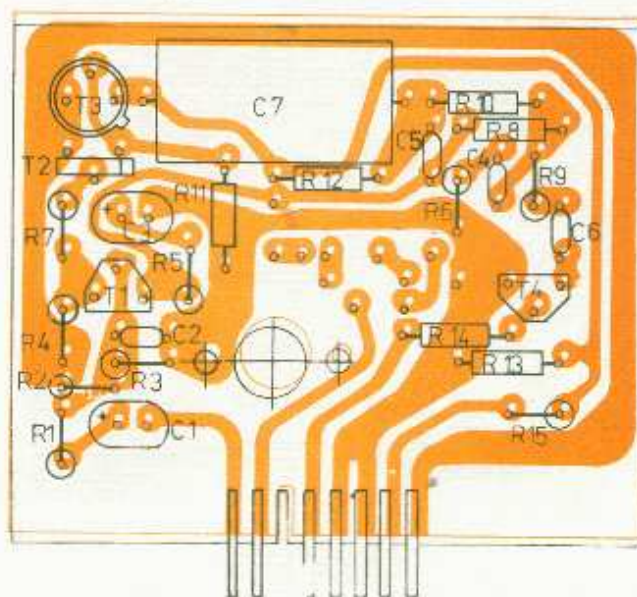
Obr. 24. Deska záznamového zesilovače (pohled ze strany součástek)
