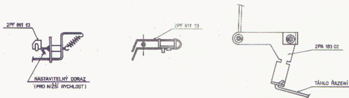
obr. 3. Nastavení řazení rychlosti
