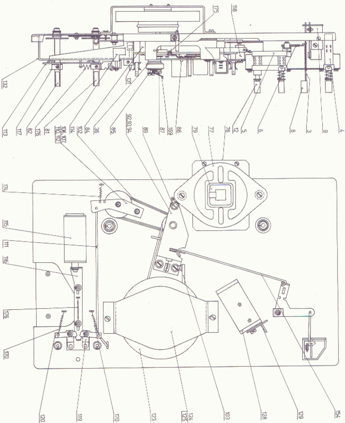
obr. 45. Náhradní díly (mechanický soustava)
