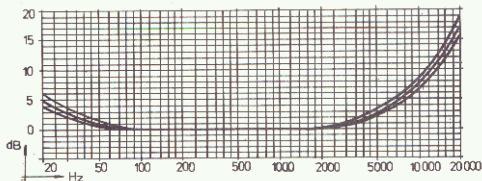
obr. 26. Kmitočtová charakteristika ZZ pro rychlost "9"
