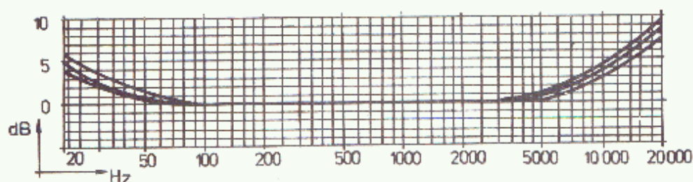
obr. 27. Kmitočtová charakteristika ZX pro rychlost "19"
