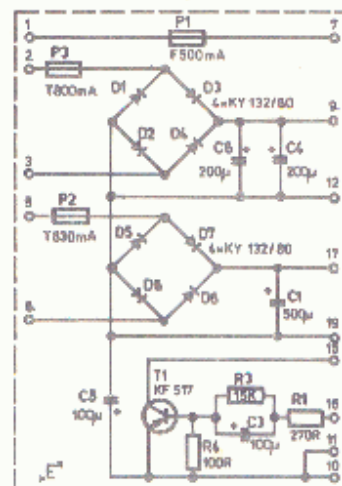
obr. 41. Schéma napájecího zdroje od v.č. 402701
