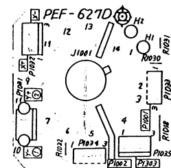
PEF-627D PCB
