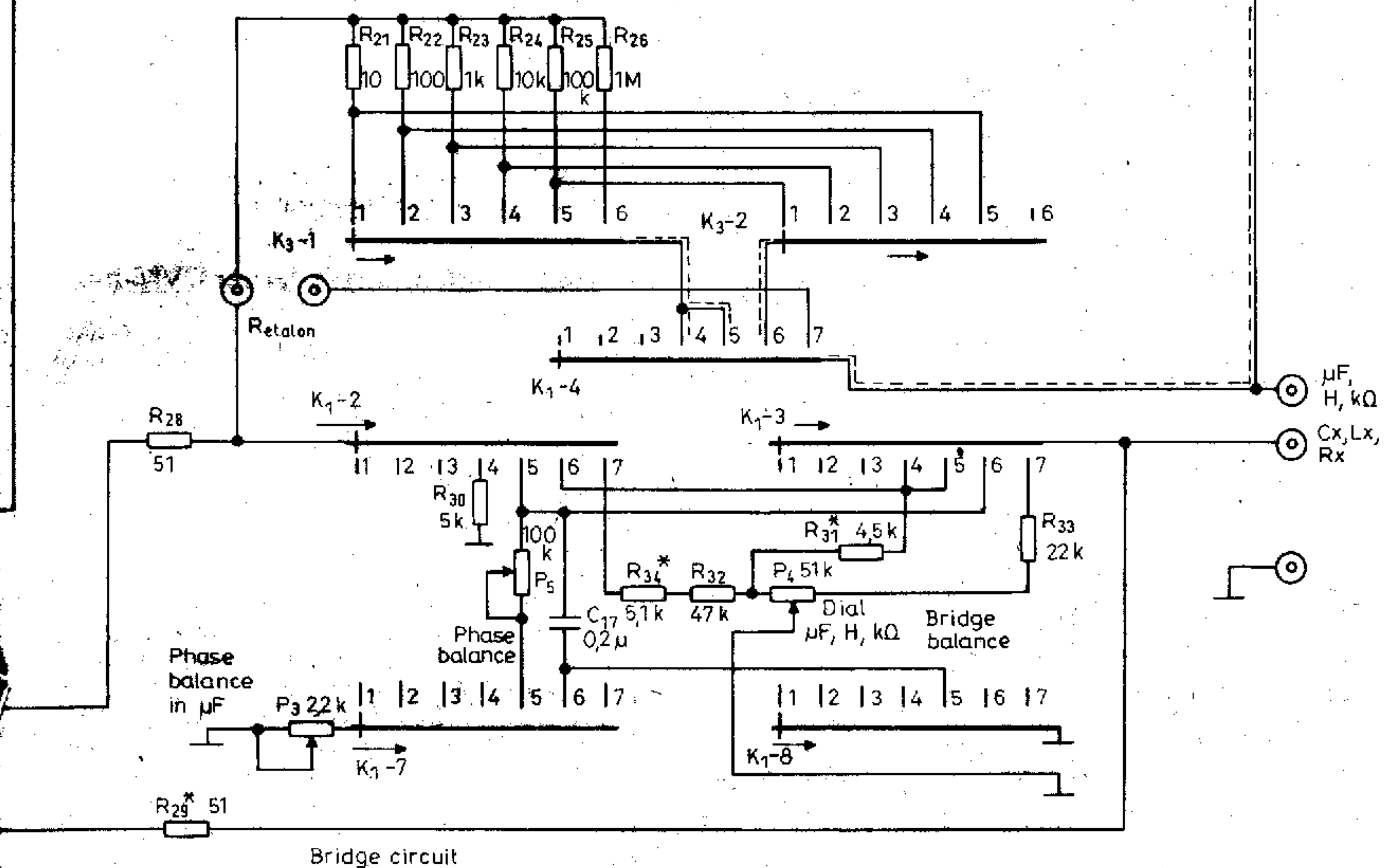
Q-52 típus. RLC f -mérő (TR 2102/A)
